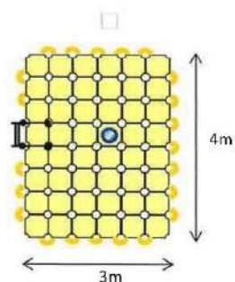
Système d'ancrage (vue de face)
